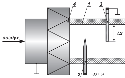
Рис. 1. Устройство для ионизации воздуха: 1 – камера из диэлектрического материала; 2 – коронирующий электрод в виде иглы; 3 – управляющий заземленный электрод, имеющий микрометрическую резьбу, которая позволяет изменять глубину его погружения в камеру устройства на глубину \Delta x ; 4 – предварительный фильтр тонкой очистки)
