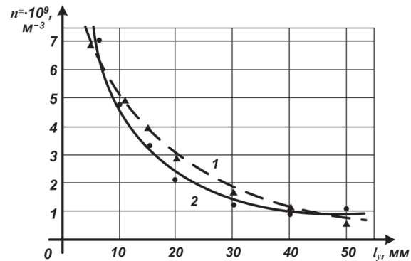
Рис. 2. Зависимость концентрации n^{\pm} лёгких аэроионов на выходе устройства для ионизации воздуха от перемещения l_y управляющего электрода: 1, \blacktriangle – отрицательные аэроионы; 2, \bullet – положительные аэроионы)
