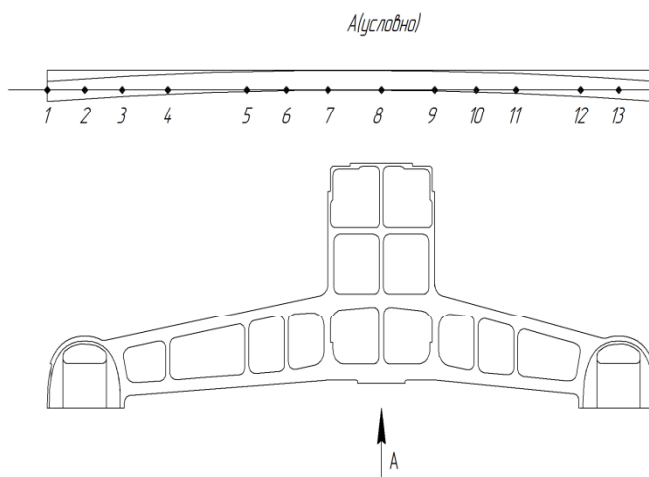
Рис. 2. Схема измерения отклонения от плоскостности в контрольных точках
