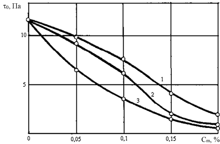
Рис. 1. Зависимость предельного напряжения сдвига суспензий C_3S при VT=0,48 от дозировки добавок: 1 – C-3; 2 – CB-3; 3 – C-3+CB-3
