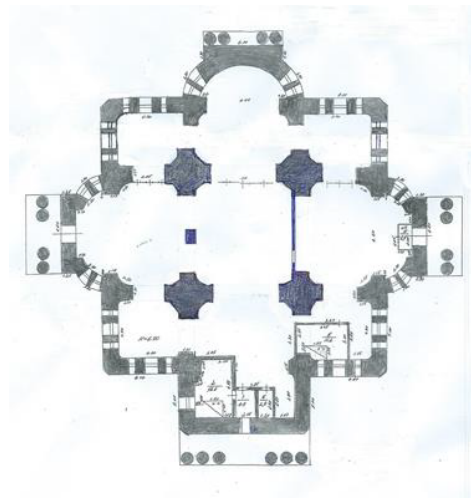
Рис. 5. План храма
