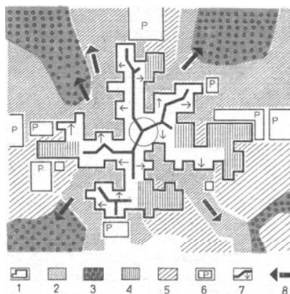
Рис. 2. Принципиальная модель взаимосвязанной системы внутригородских и пригородных открытых пространств: 1 – селитебные территории; 2 – зеленые клинья открытых пространств – головные зоны рекреации; 3 – экологическая зона; 4 – промышленные и коммунально-складские территории; 5 – открытые пространства коммунально-хозяйственного назначения; 6 – зоны градостроительного развития; 7 – условная линия, разделяющая селитебные территории на районы тяготения к открытым пространствам; 8 – сохраняемые непрерывные связи городских и загородных открытых пространств [3]
