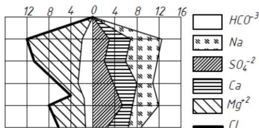
Рис. 2 Состав водной вытяжки из лёссового грунта
