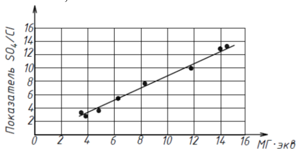
Рис. 1 Прямолинейная зависимость показателей SO 4 /Cl и Na/Cl в водной вытяжке
