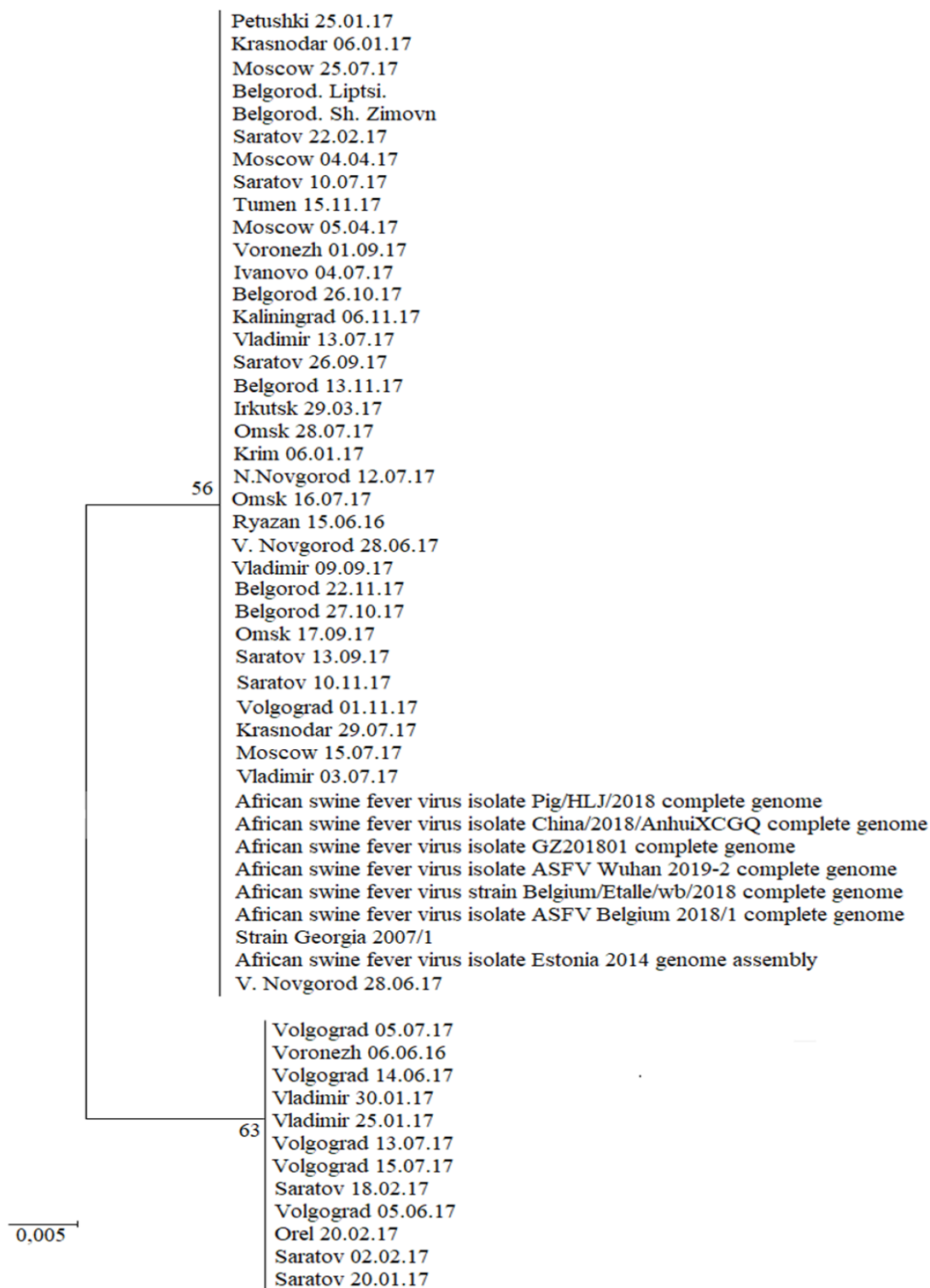
Рис. 1 – Филогенетическое древо, построенное по методу «Bootstrap (максимального правдоподобия)» на основании данных нуклеотидных последовательностей В602L изолятов вируса АЧС, выделенных на территории РФ с 2016 г. по 2019 г.
