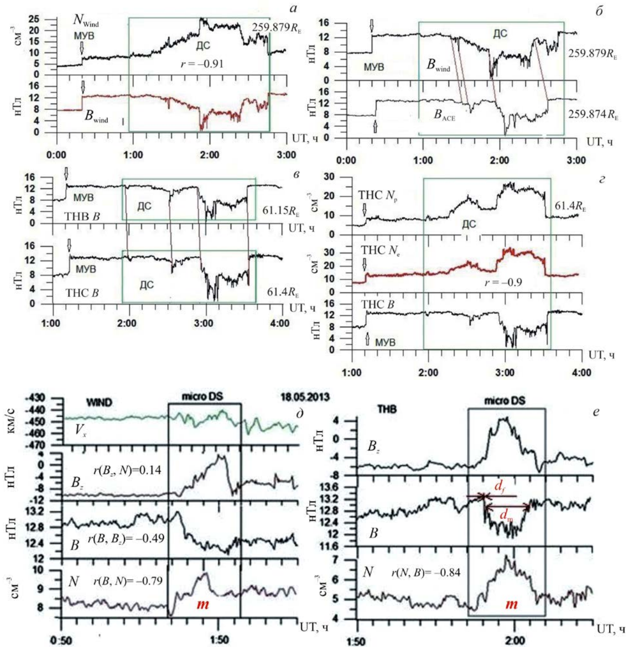
Рис. 4. Распространение ДС в солнечном ветре: a — вариации концентрации СВ ( N ) и модуля ММП ( B ) по данным Wind; б — вариации модуля B ММП по данным Wind и ACE; в — вариации модуля B ММП на спутниках ТНВ и ТНС вблизи орбиты Земли (прямые линии соединяют характерные детали для определения запаздывания); г — вариации модуля B ММП, концентрации протонов и электронов по данным ТНС вблизи орбиты Земли (справа указано расстояние в R_E соответствующего спутника от центра Земли в момент измерений). Данные получены на сайте [ http://cdaweb.gsfc.nasa.gov/cgi-bin/eval2.cgi ]. Сохранение микроструктуры m ДС на больших расстояниях от Солнца: д — параметры СВ и ММП на орбите Wind; е — тот же участок СВ на орбите ТНВ вблизи Земли
