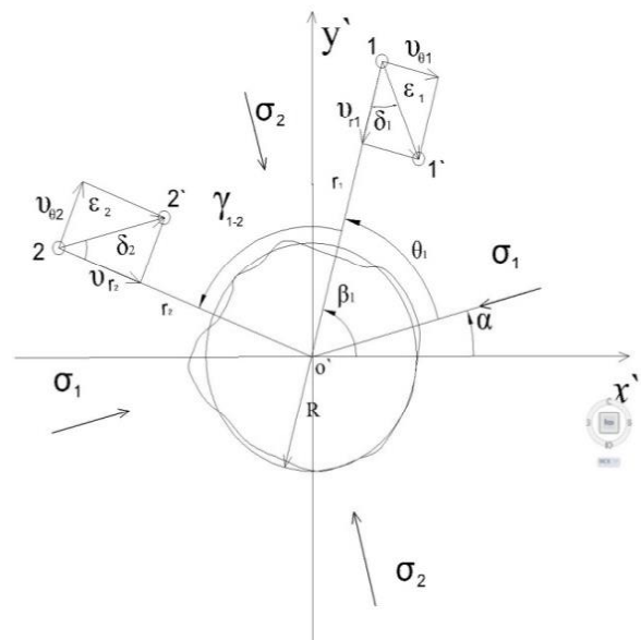
Рис. 4. Схема для расчета напряжений при выходе зоны обрушения на земную поверхность в виде окружности
