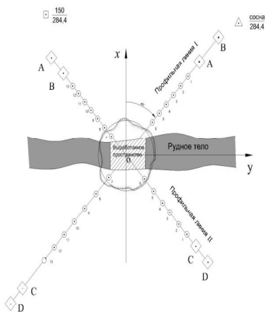
Рис. 2. Схема расположения профильных линий под углом 45° к простиранию рудного тела
