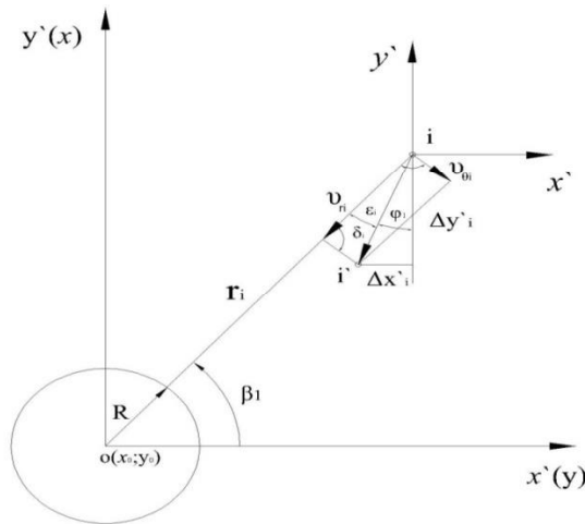
Рис. 3. Схема смещения рабочего i -го репера после выхода зоны обрушения на земную поверхность
