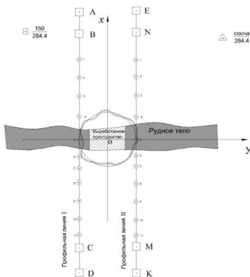
Рис. 1. Схема расположения профильных линий вкрест простирания рудного тела
