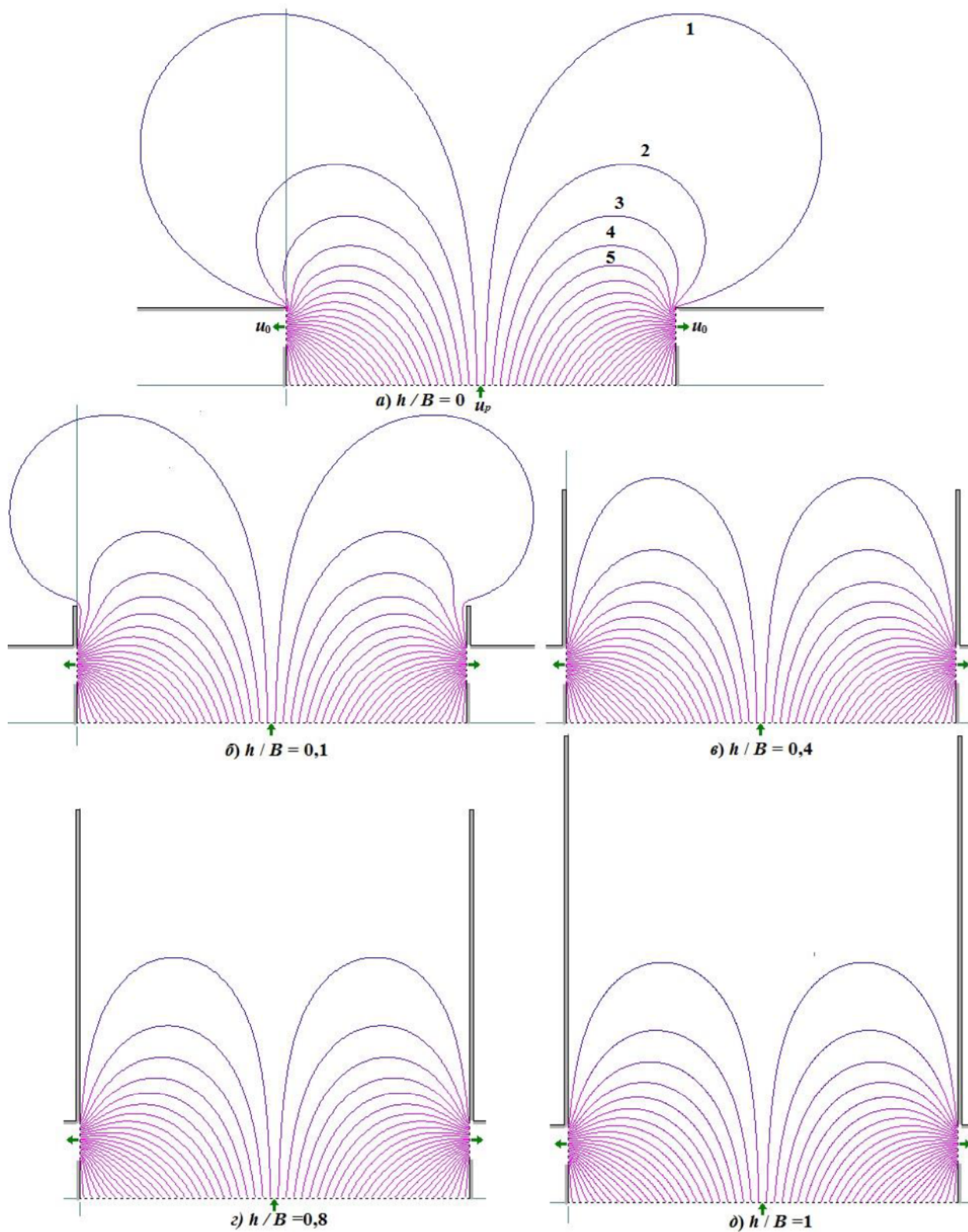
Рис. 3. Линии тока вблизи двубортового отсоса при разных высотах механического экрана
