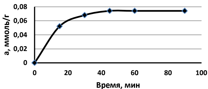
Рис. 1 Влияние времени контакта модельного раствора соли кадмия ( C_0 = 8 \cdot 10^{-3} моль/л) и лишайника кладония лесная ( Cladonia sylvatica ) на сорбцию ионов кадмия (II)
