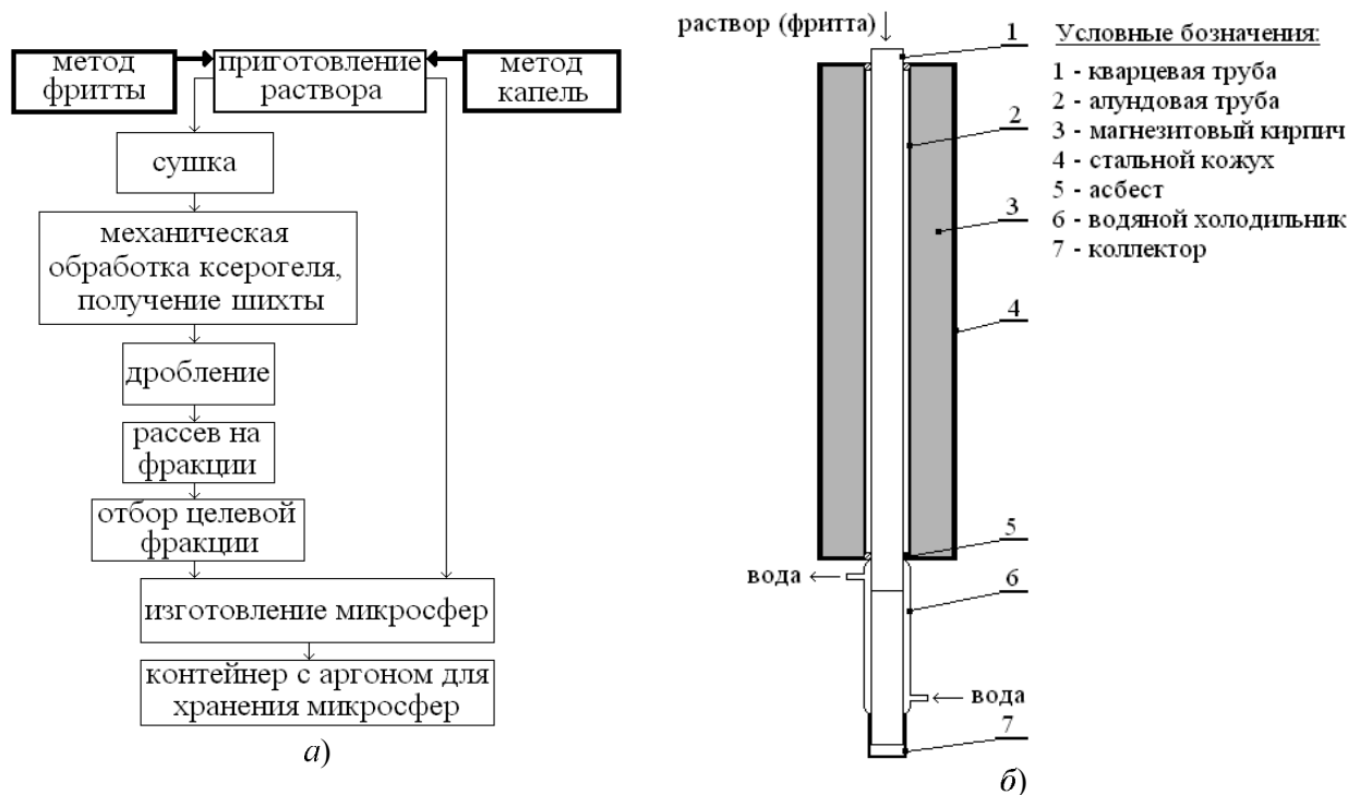
Рис. 1. Технологическая схема изготовления стеклянных микросфер:
