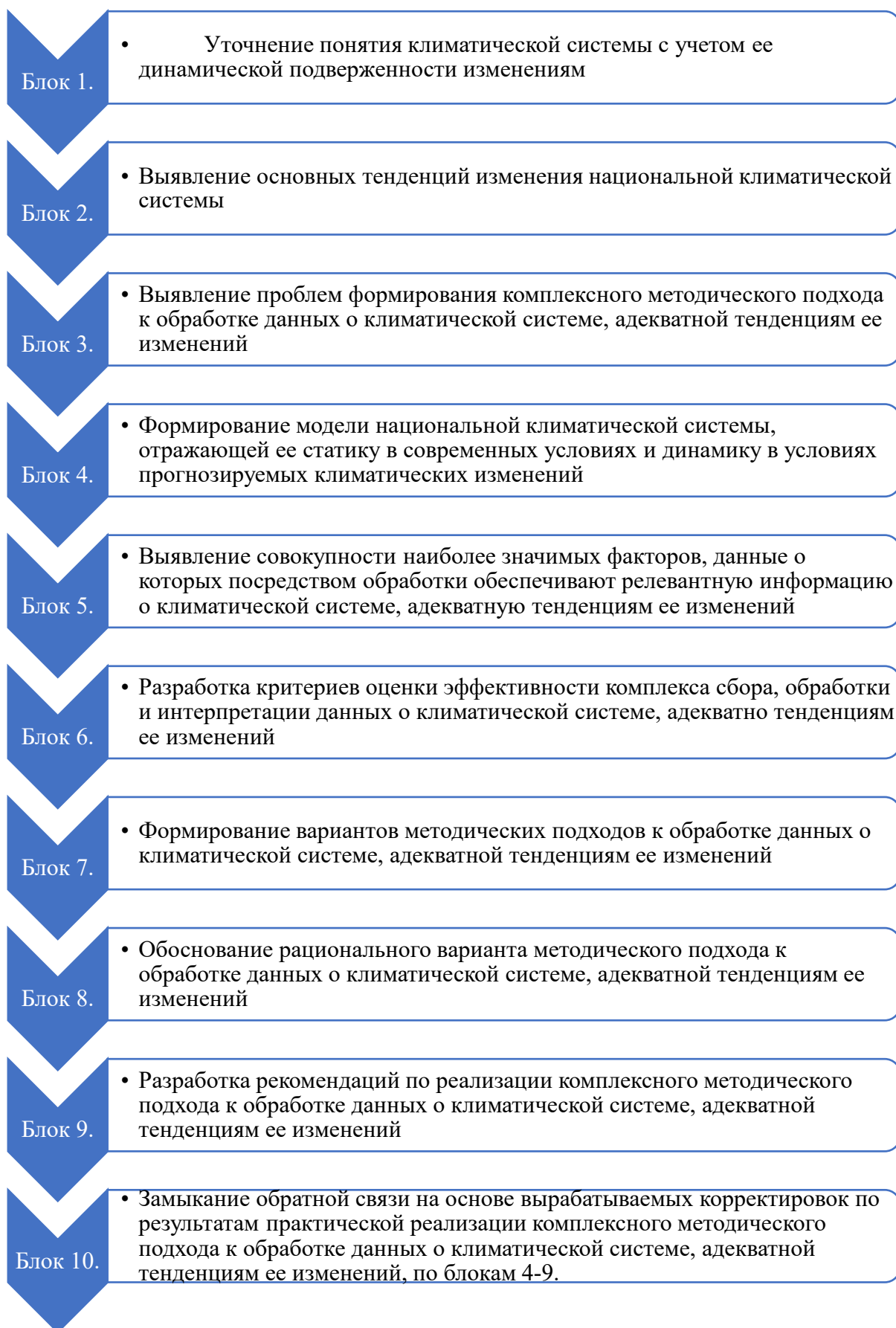
Рис. 1. Алгоритм решения проблемы формирования комплексного методического подхода к обработке данных о климатической системе, адекватной тенденциям ее изменений
