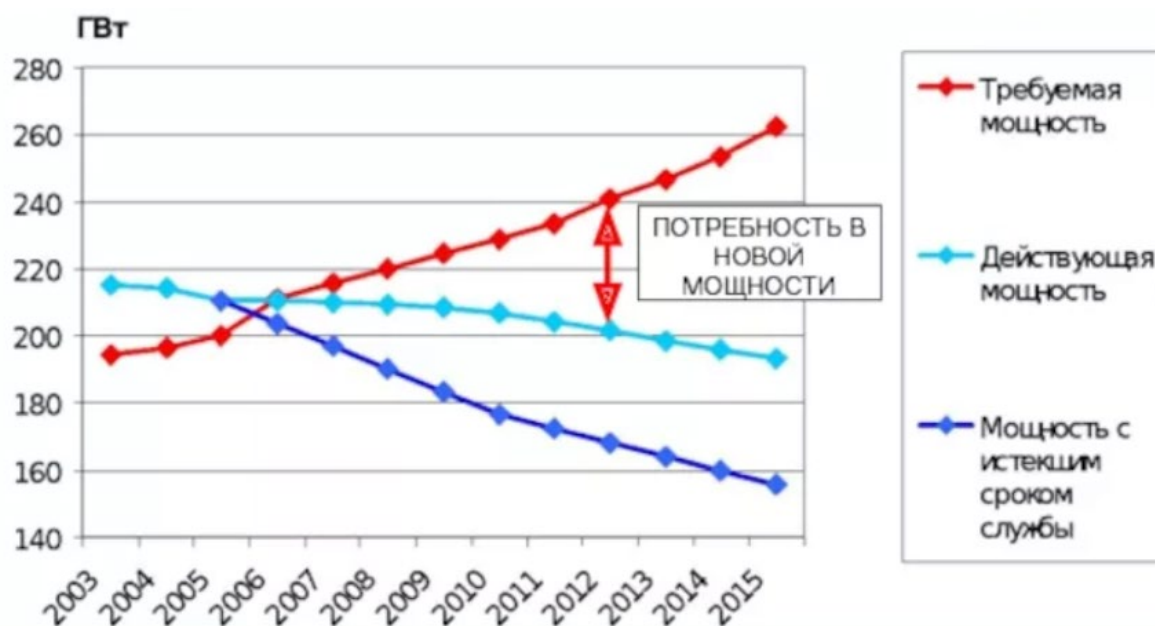
Рис. 9. «Крест Чубайса» по данным ИНЭИ РАН, демонстрирующий как требуемые мощности электроэнергетики стали существенно превосходить действующие
