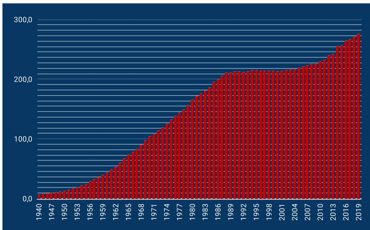
Рис. 7. Установленная мощность-брутто электростанций России, 1940—2019 гг. (по данным Росстата), млн кВт. [4]
