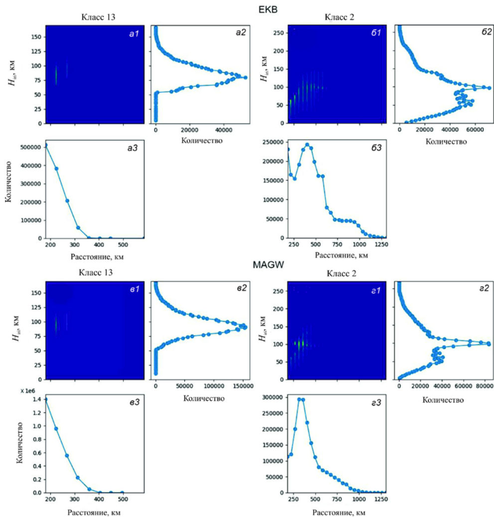
Рис. 5. Сравнение высотно-дальностных распределений классов 13 и 2 за период январь 2021 – март 2022 г.: a1–e1 — высотно-дальностное распределение частоты наблюдения следов; a2–e2 — частота появления рассеивателей в зависимости от высоты, рассчитанной по траектории распространения сигнала; a3–e3 — распределение сигналов как функция радиолокационной дальности
