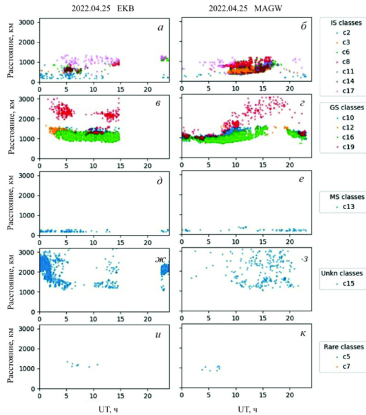
Рис. 3. Пример работы алгоритма на данных радаров ЕКВ (слева) и MAGW ИСЗФ СО РАН (справа) 25 апреля 2022 г. Сверху вниз: классы типа ионосферных рассеяний (а, б); классы типа рассеяния от земной поверхности (в, г); классы типа метеорного рассеяния (д, е); неидентифицированные классы (ж, з); редко наблюдаемые классы (и, к)
